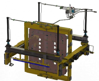
Geschlossenes Befüll-System der Schliesseinheit (AO) -kein Sandaustrocknen-
