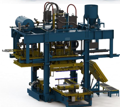
Geteilte Versorgung von Katalysator und Spülluft (patentiert)
