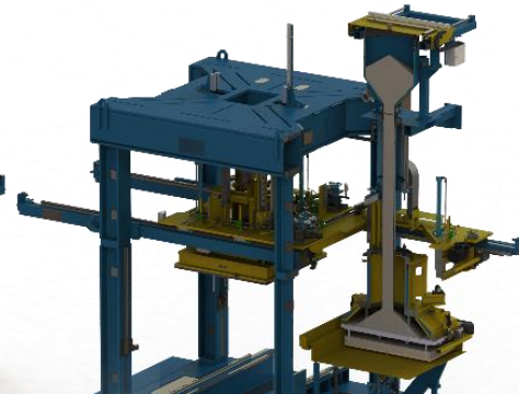
Geschlossenes Befüll-System der Schliesseinheit (AO) -kein Sandaustrocknen-
